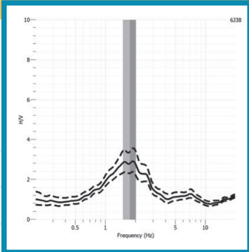
Figura 22. Comportamiento vibracional en cercanías a la ECAMP (fuente: INGEMMET).
