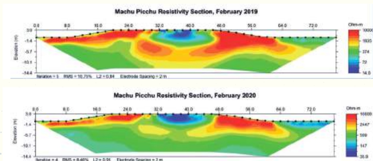
Figura 20. Comparación del permafrost (color rojo) en la ECAMP (fuente: INGEMMET).
