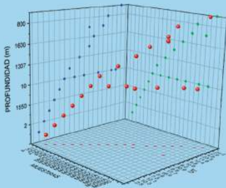
Figura 8. Distribución espacial de las unidades tritadas de tritio a diferentes profundidades. (Fuente: IPEN).
